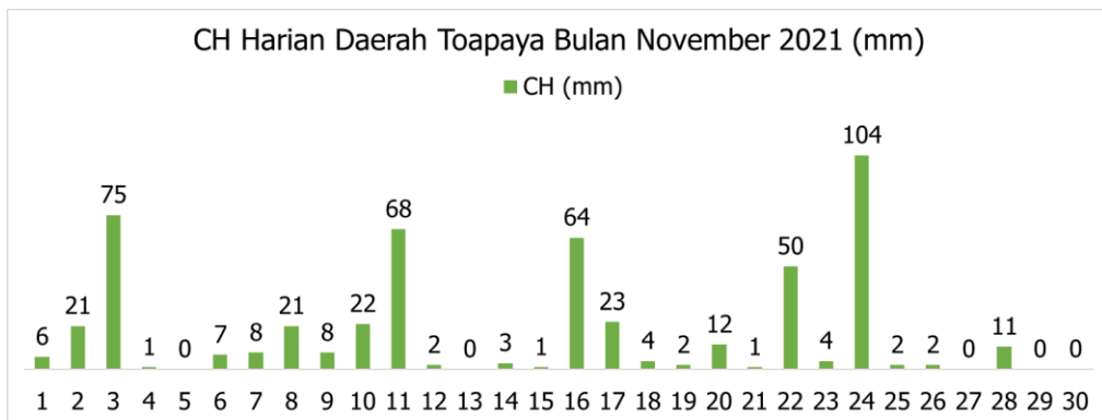
Gambar 73. Curah hujan harian bulan (a) September, (b) Oktober, dan (c) November 2021 (BMKG, 2021)
